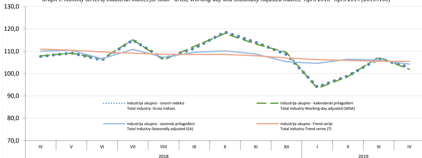
Grafik 1. Mjesečna serija indeksa industrija ukupno - izvorni, kalendarski i sezonski prilagođeni indeksi: travanj 2018 - travanj 2019 (2015=100) Graph 1. Monthly series of industrial indices for total - Gross, Working-day and Seasonally Adjusted indices: April 2018 - April 2019 (2015=100)
