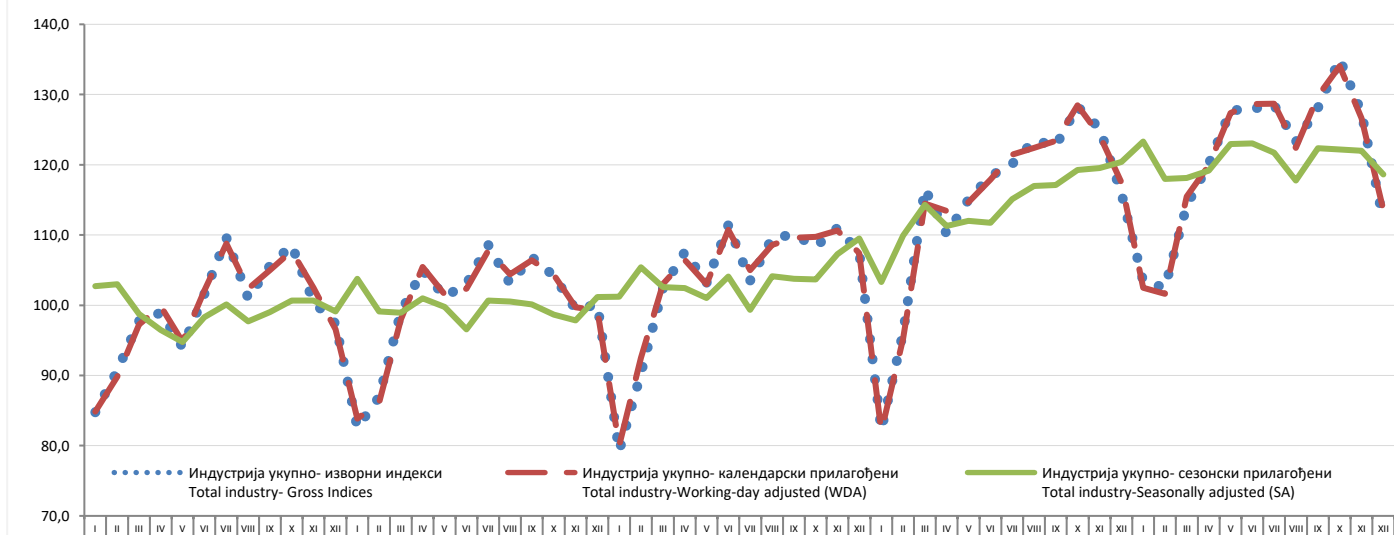
График 1. Временска серија индустрија укупно - изворни, календарски и сезонски прилагођени индекси: јануар 2014 - децембар 2018 (2015 = 100) Graph 1. Time series for total industry - Gross, Working-day and Seasonally Adjusted indices: January 2014 - December 2018 (2015=100)
