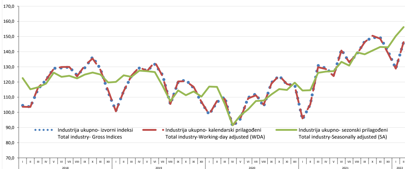
Grafik 1. Vremenska serija industrija ukupno - izvorni, kalendarski i sezonski prilagođeni indeksi: januar 2018 - februar 2022 (2015=100) Graph 1. Time series for total industry - Gross, Working-day and Seasonally Adjusted indices: January 2018 - February 2022 (2015=100)
