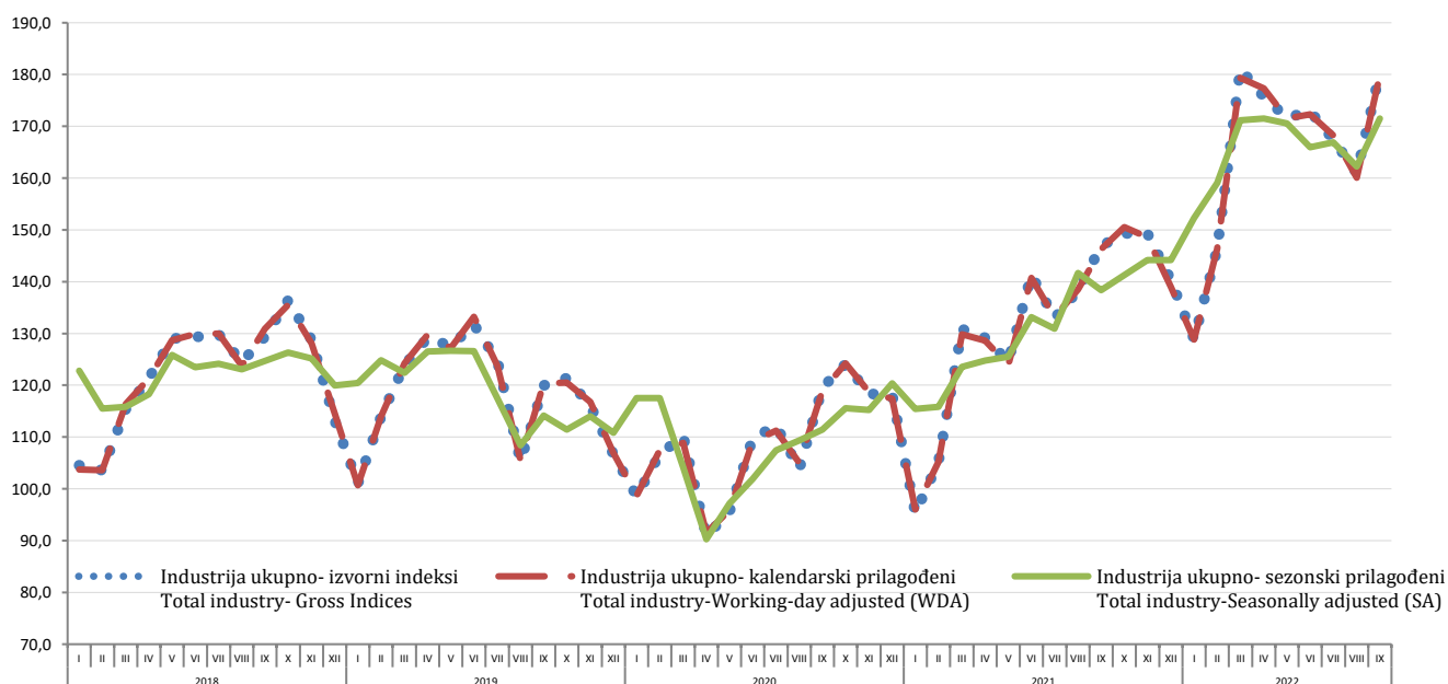
Grafik 1. Vremenska serija industrija ukupno - izvorni, kalendarski i sezonski prilagođeni indeksi: siječanj 2018 - rujna 2022 (2015=100) Graph 1. Time series for total industry - Gross, Working-day and Seasonally Adjusted indices: January 2018 - September 2022 (2015=100)
