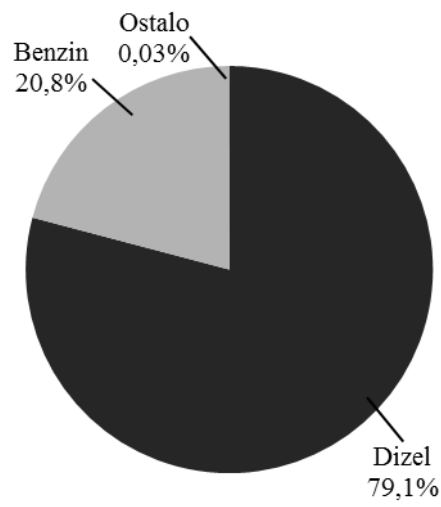
G. 2. Prvi put registrirana putnička motorna vozila po tipu pogonske energije za 2012. godinu G. 2. First time registered passenger motor vehicles by type of motor energy for 2012 year
