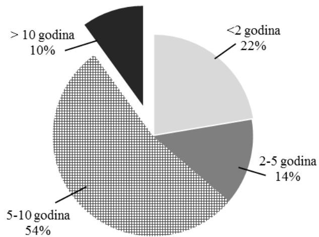
G.3. Prvi put registrirana cestovna motorna vozila po godinama starosti za 2012. godinu G.3. First time registered road motor vehicles by age for 2012 year
