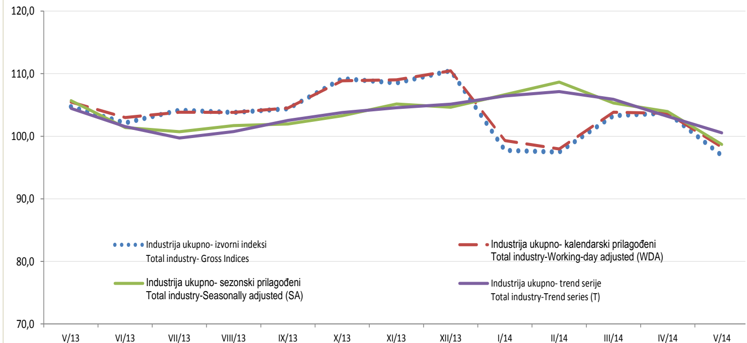
Grafik 1. Mjesečna serija indeksa industrija ukupno - izvorni, kalendarski i sezonski prilagođeni indeksi: maj 2013 -maj 2014 (2010 = 100) Graph 1. Monthly series of industrial indices for total - Gross, Working-day and Seasonally Adjusted indices: May 2013 - May 2014
