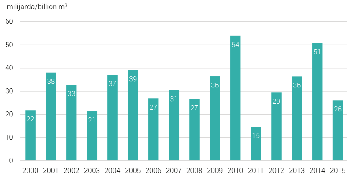
Grafikon 24. Obnovljivi slatkovodni resursi, 2000 – 2015. Graph 24. Renewable freshwater resources, 2000 - 2015
