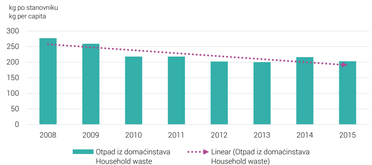
Grafikon 7. Količine nastalog otpada iz domaćinstava Graph 7. Quantities of generated household waste
