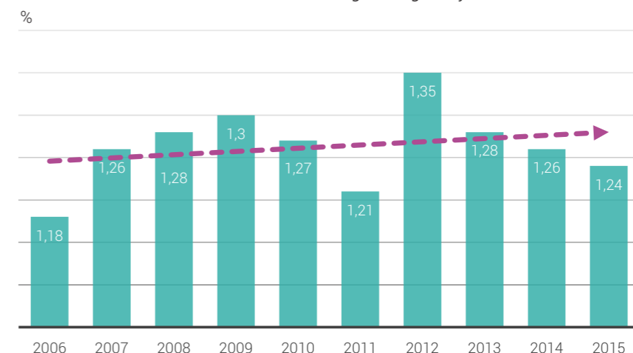
Grafikon 14. Ukupna stopa fertiliteta, korisnici, % Graph 14. Total fertility rate, %
