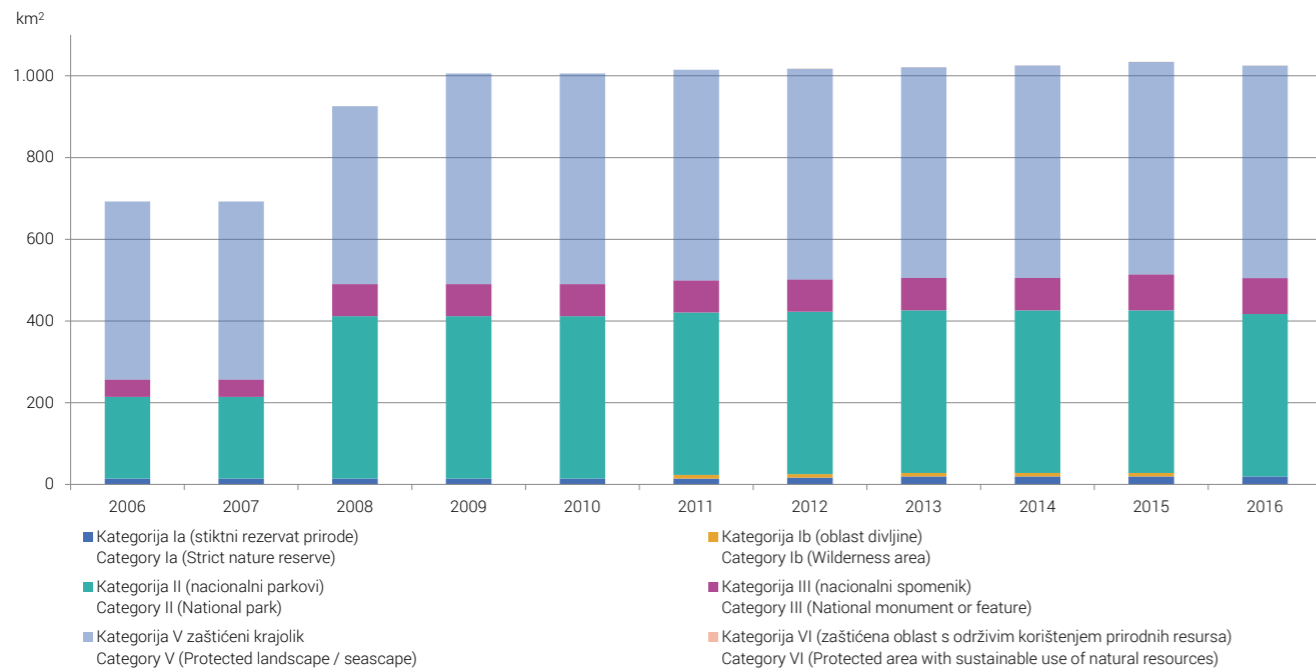
Grafikon 22. IUCN kategorije zaštićenih područja 2006 – 2016, km² Graph 22. IUCN Designated areas 2006 – 2016, km²
